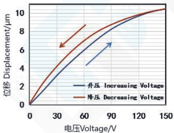
位移 Displacement(9N/20°C)
