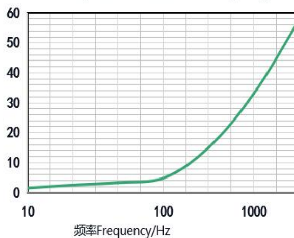
温升 & 频率变化图 Temperature Rise vs. Drive Frequency
